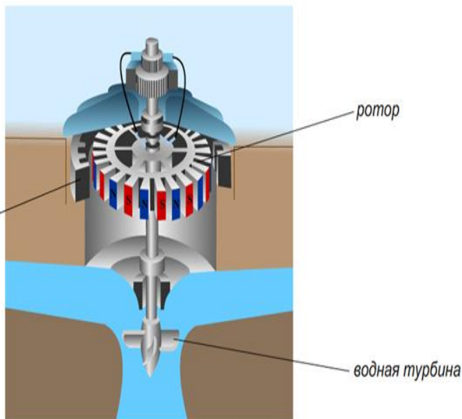
Рисунок 3.9. Работа гидрогенератора
