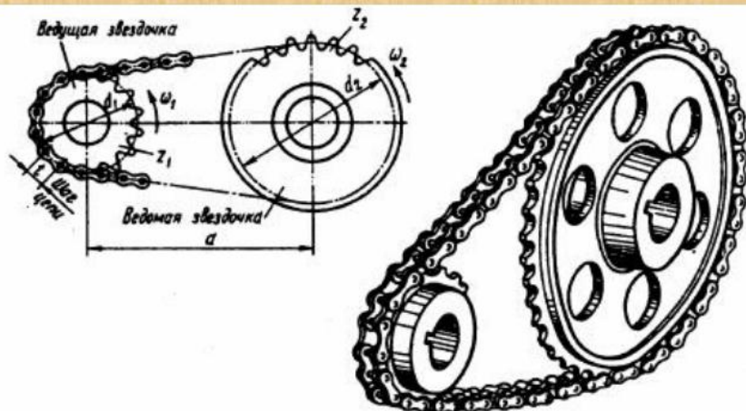
Цепная передача
